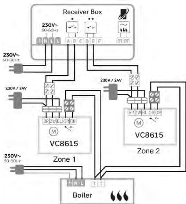
Cablaggio 2 valvole di zona 824V) e bollitore on/off (24V)
